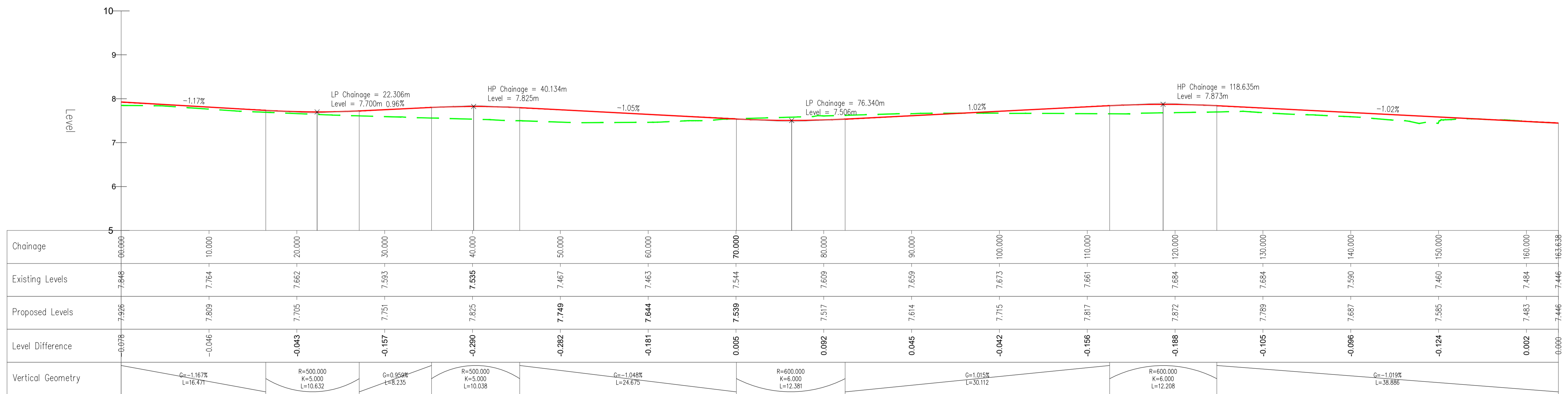
ROAD 2. SCALE: H=1:250; V=1:50; DATUM: 5.000
