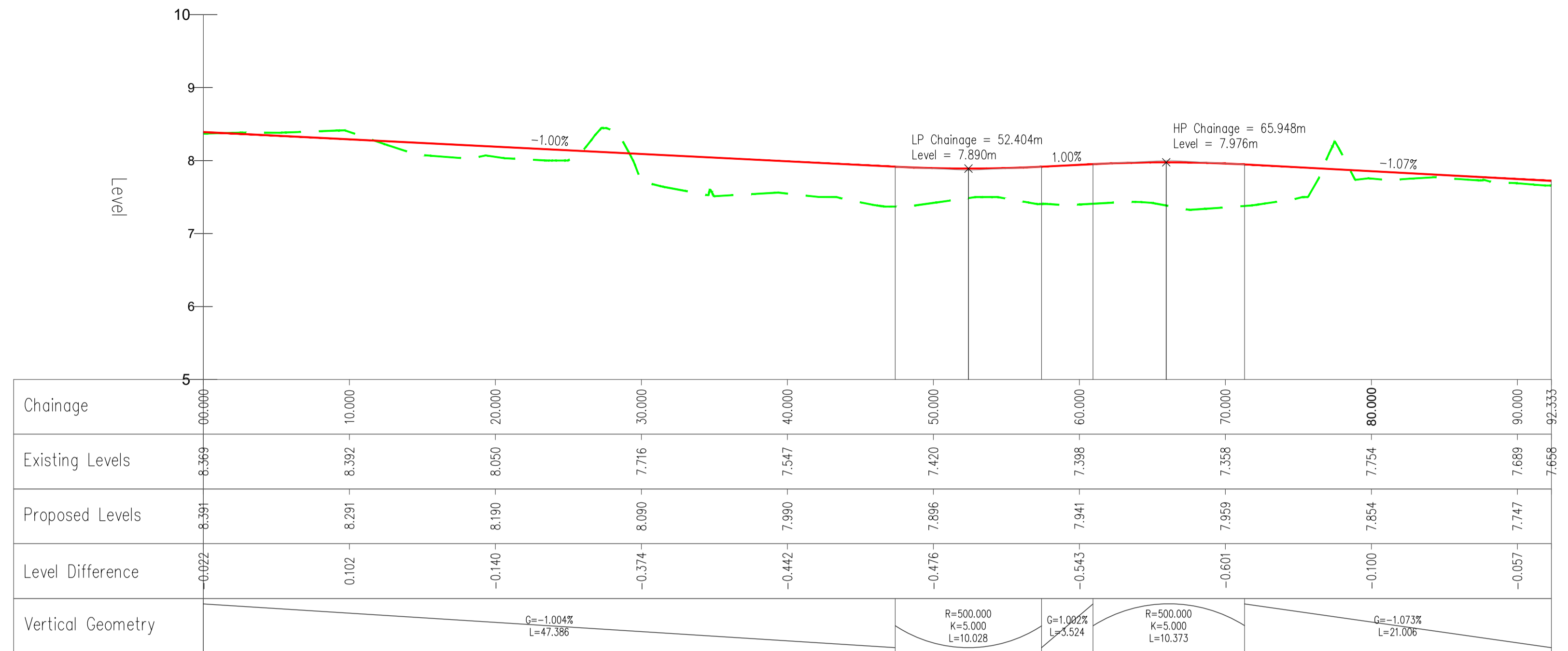
ROAD 3. SCALE: H=1:250; V=1:50; DATUM: 5.000
