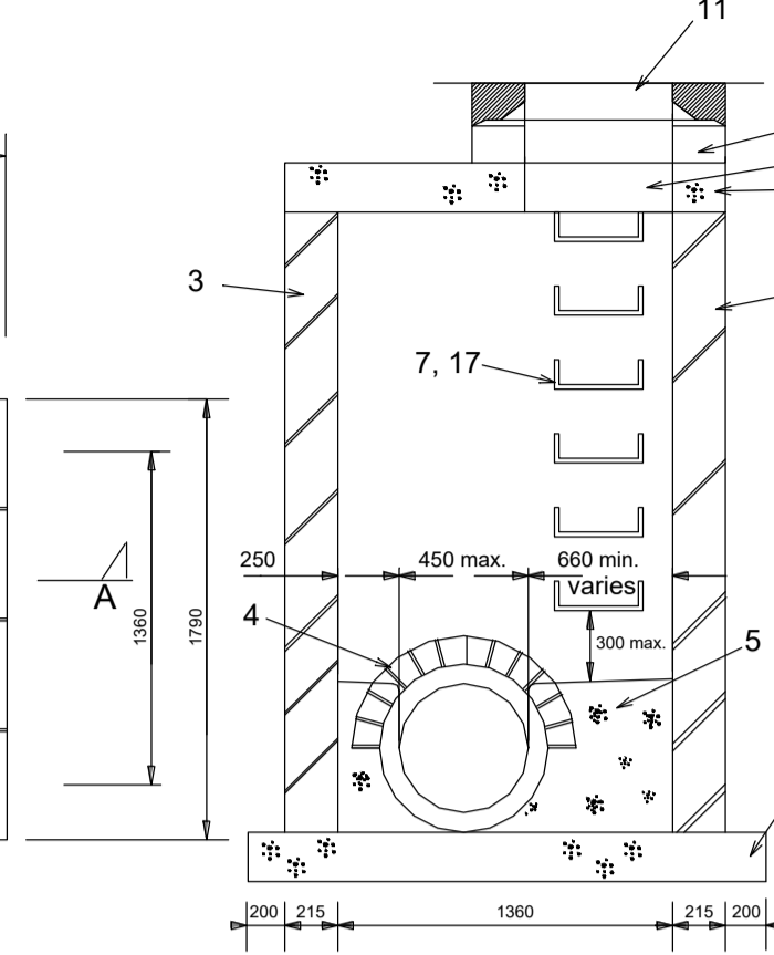
Section A-A
