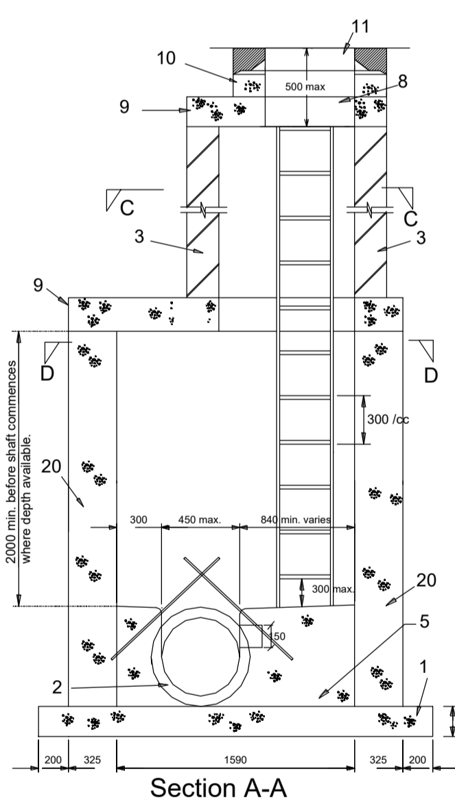
Section A-A
